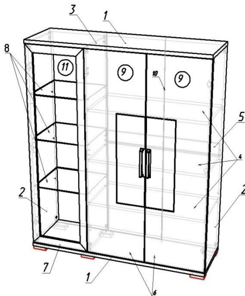
Рис.1 Схема сборки
